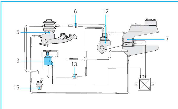
Figure 3 AGR-System (mit mech. Druckwandler) EGR-System (with mech. pressure transformer) Système de recyclage (avec convertisseur de pression) Sistema de recirculación (con convertidor de presión) Sistema de ricirculazione (con convertitore di pressione)
