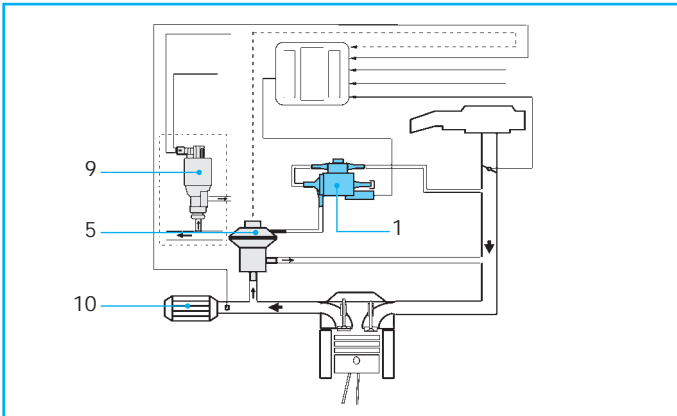
Figure 2 AGR-System (Otto-Motor) EGR-System (Otto Engine) Système de recyclage (moteur à essence) Sistema de recirculación (motor de gasolina) Sistema de ricirculazione (motore a benzina)
