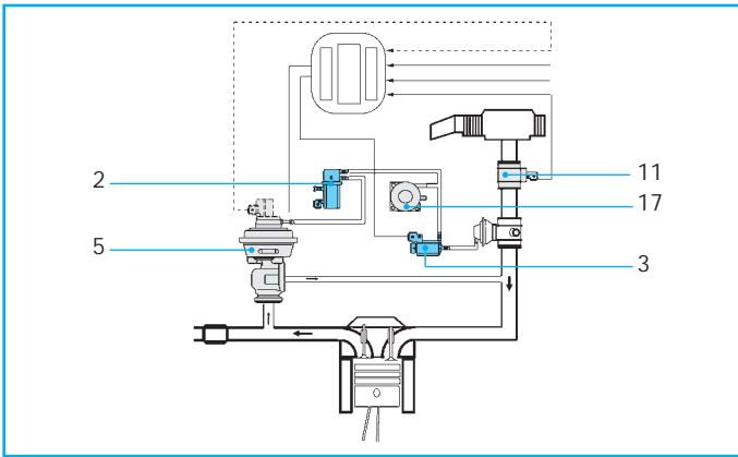
AGR-Systeme EGR-systems Systèmes de recyclage des gaz Sistemas de recirculación de gases Sistemi de ricirculazione dei gas di scario (Fig. 1, 2, 3)
